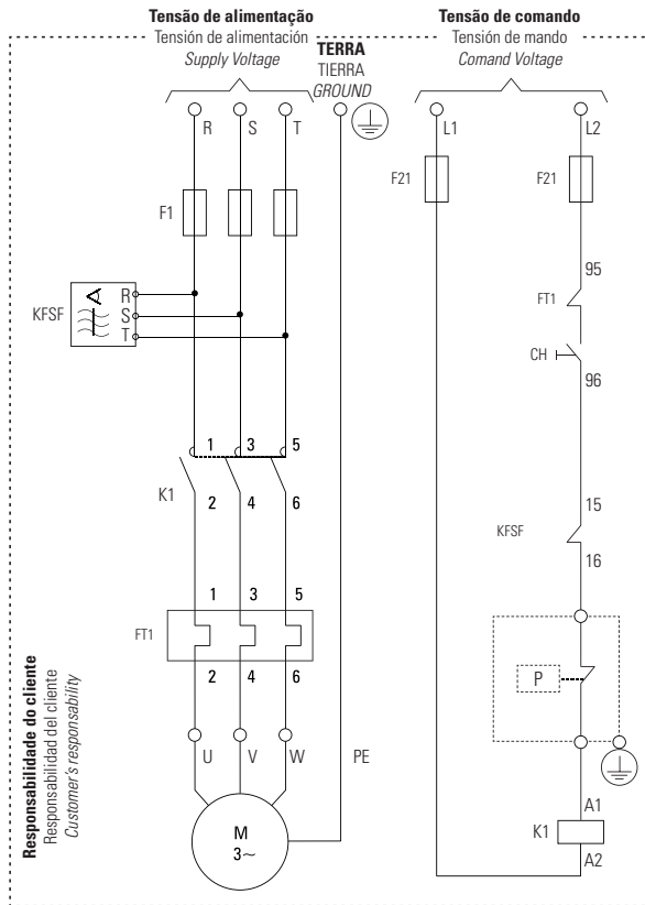
MOTORES TRIFÁSICOS - PARTIDA DIRETA MOTORES TRIFÁSICOS - PARTIDA DIRETA THREE-PHASE MOTOR WITH DIRECT STARTER
